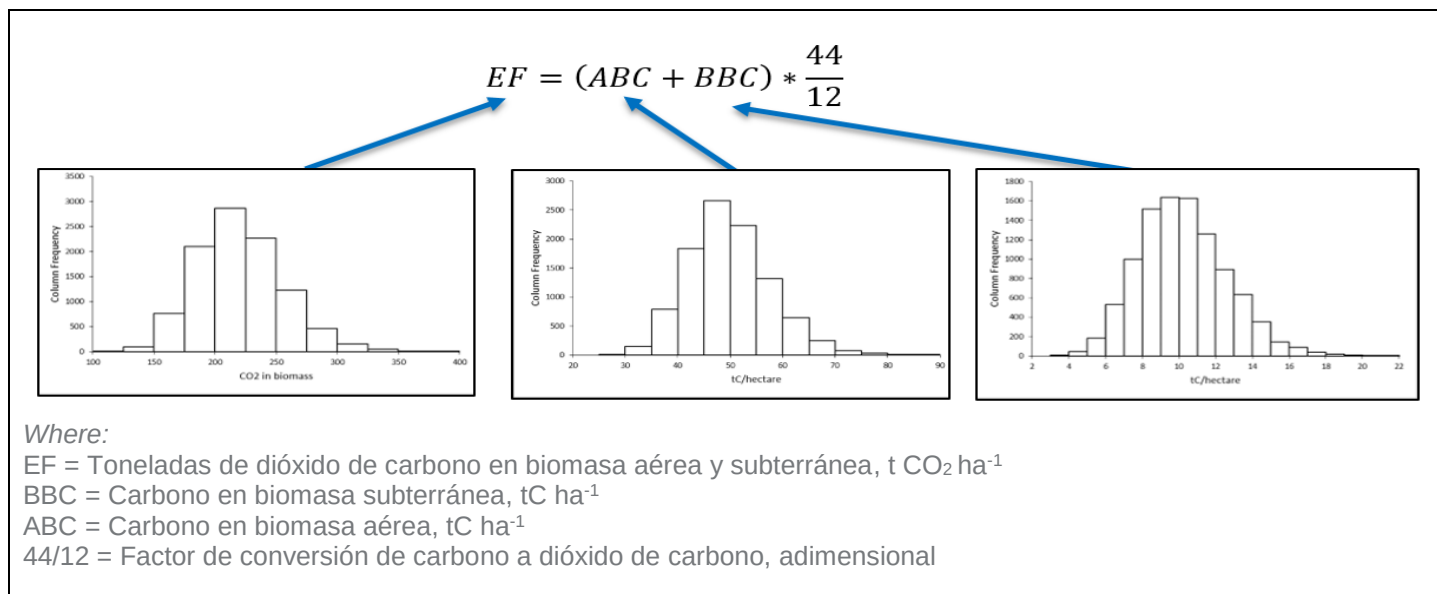
Figure A7. Cálculo de la distribución del factor de emisión en base a las distribuciones de biomasa aérea y subterránea
