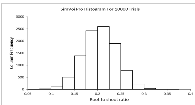
Figure A5. Simulación Monte Carlo de la relación raíz:vástago
