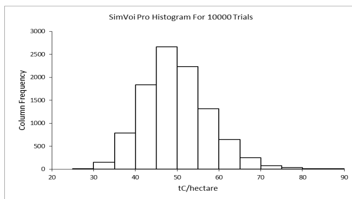
Figure A4. Simulaciones de Monte Carlo truncadas con un valor máximo de 90 toneladas de carbono en biomasa aérea por hectárea
