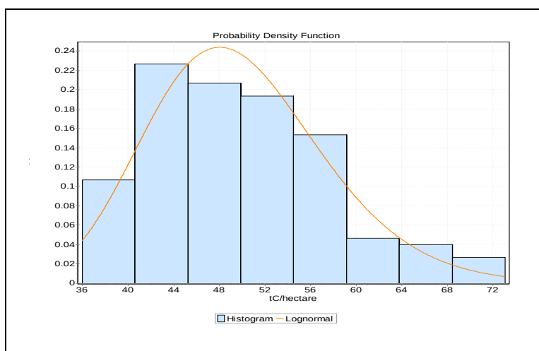
Figure A2. Distribución lognormal ajustada a los datos de biomasa aérea
