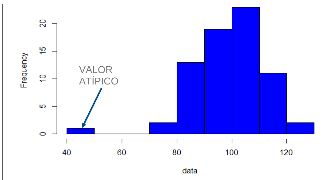
Figura 4. Ilustración de datos atípicos
