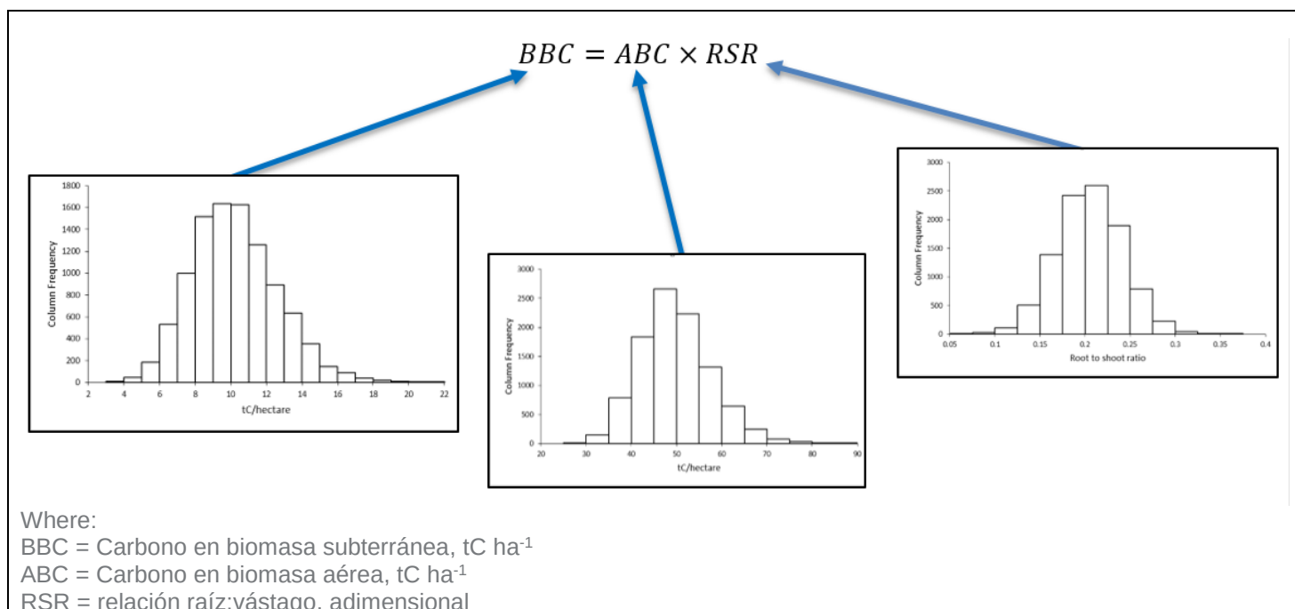
Figure A6. Aplicación de simulaciones de Monte Carlo en la ecuación para identificar la distribución de probabilidad del contenido de carbono en la biomasa subterránea
